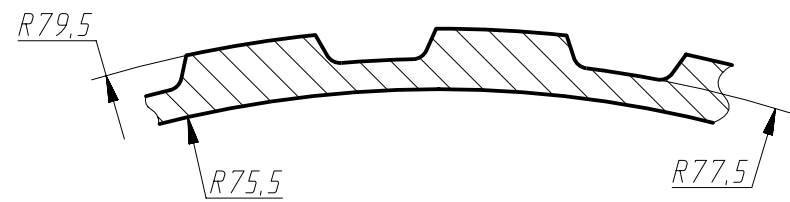
Б-Б (1:1) Редра жесткости
