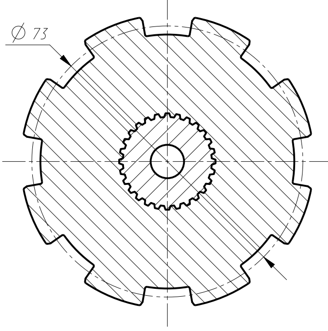
Ж-Ж (1:1)
