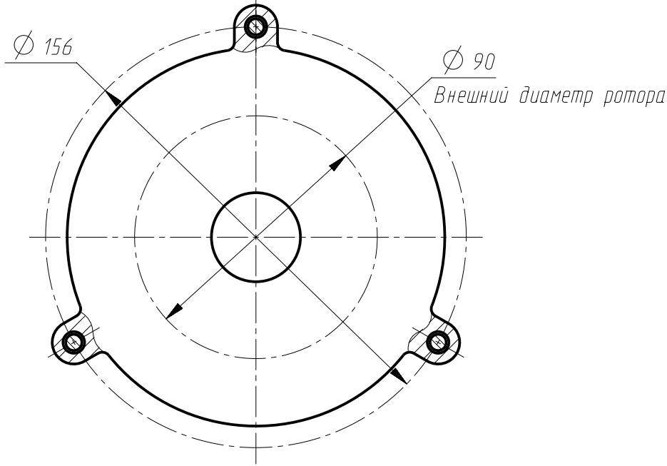
И-И (1:2)
