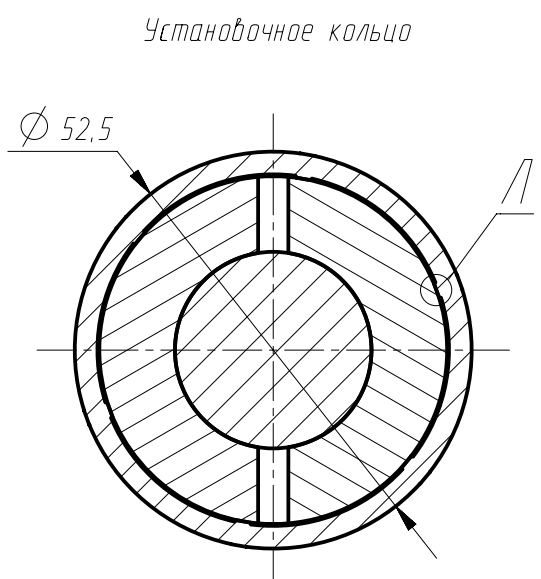
Е-Е (1:1)
